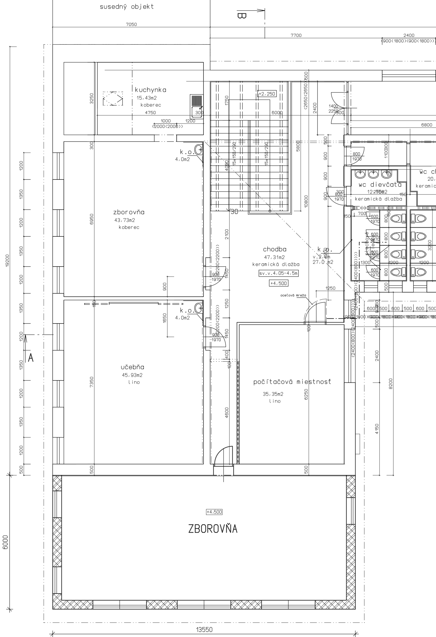
PÔDORYS POSCHODIA
